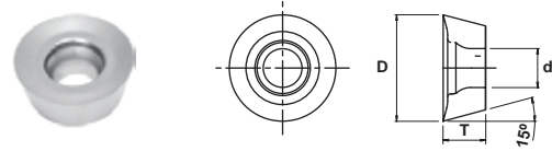
Рис.2 Полированные пластины для обработки алюминия
