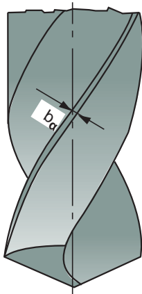
Рис.3. Ширина ленточки b_{\alpha}
