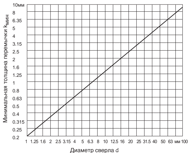
Рис.2. Толщина перемычки k_{мин}
