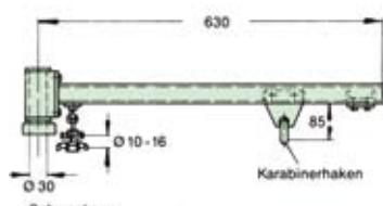
Abb. 2 Zusatzschwenkarm
